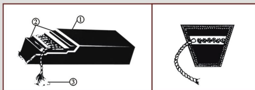
结构图 Configuration
